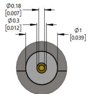
DETAIL B(20:1)
