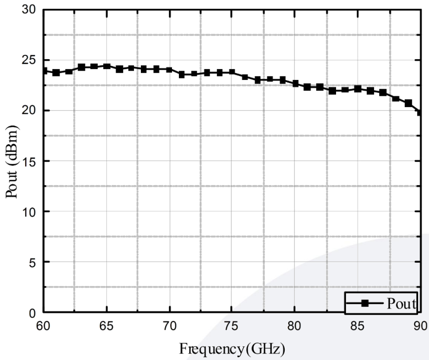
输出功率VS频率
