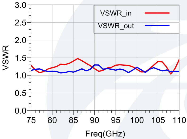
输入/输出驻波 vs. 频率
