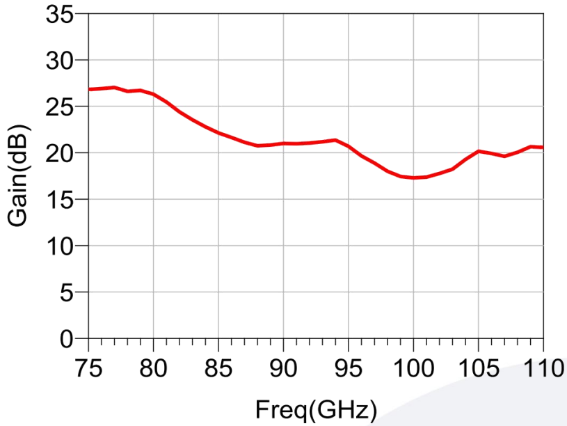
小信号增益 vs. 频率
