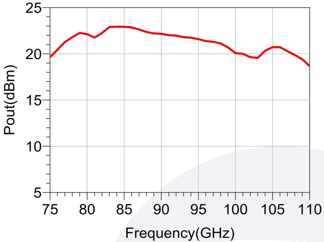
饱和输出功率 vs. 频率 @ Pin=2dBm
