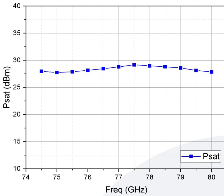
饱和输出功率VS频率
