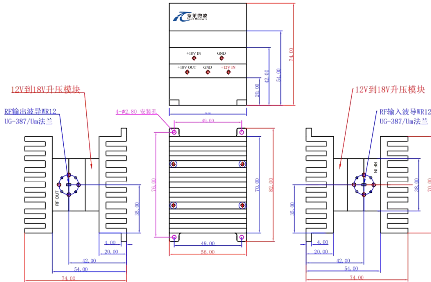
76~81GHz 26dBm 功率放大器外形图 (12V供电版本)
